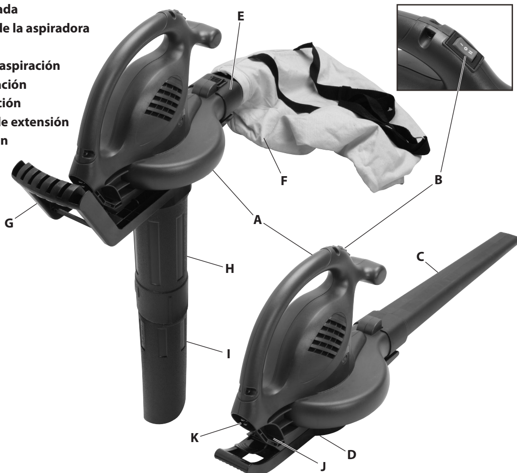
Figura 2-1: Sopladora/aspiradora eléctrica Remington®
